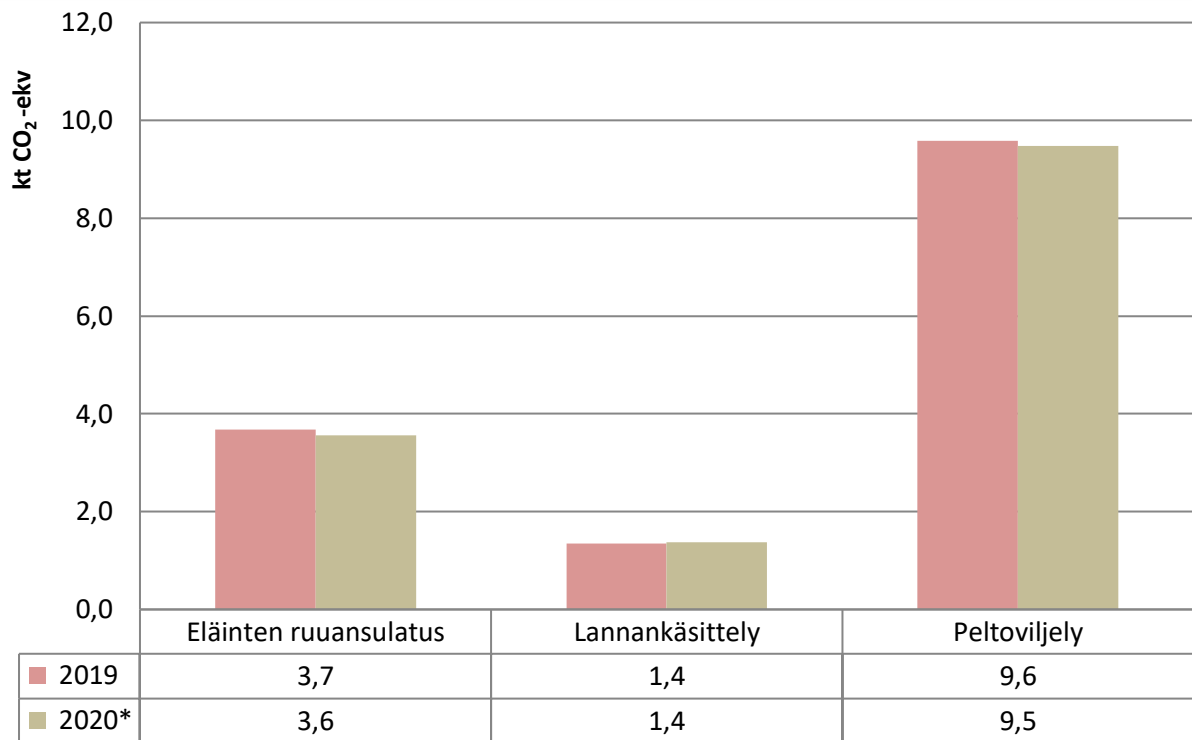
Kuva 10. Maatalouden päästöjen kehitys Orivedellä vuosina 2019–2020 jaettuna eläinten ruuansulatukseen, lannankäsittelyyn ja peltoviljelyyn päästöihin.
