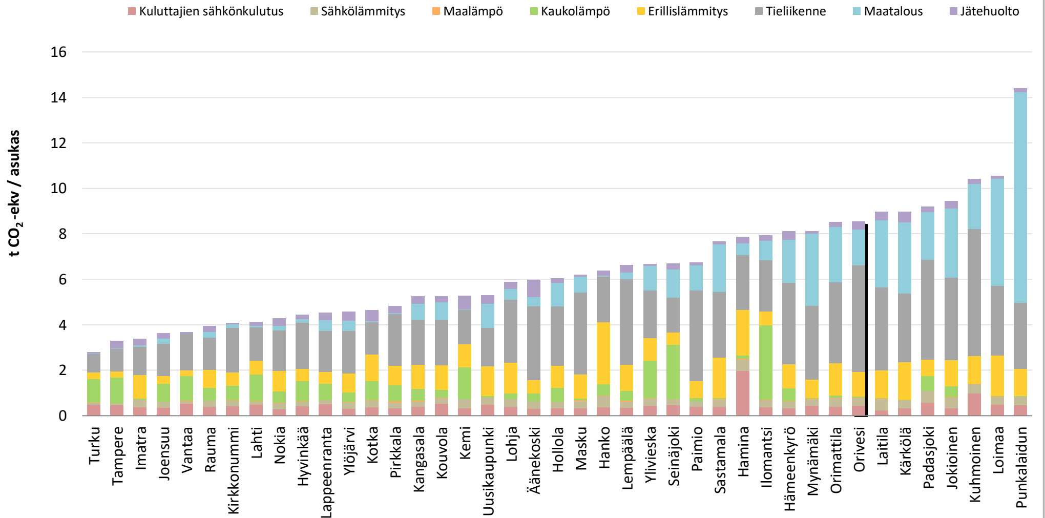
Kuva 20. CO2-raportissa mukana olevien Hinku-kuntien asukaskohtaiset päästöt sektoreittain vuonna 2019. Teollisuuden päästöt eivät ole mukana tarkastelussa.
