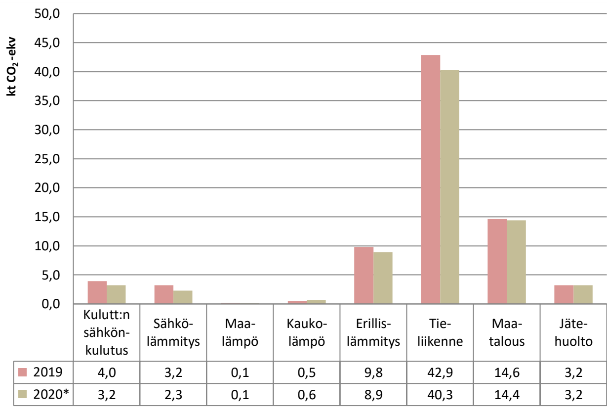
Kuva 14. Päästöt sektoreittain Orivedellä vuosina 2019–2020 ilman teollisuutta. Vuoden 2020 tieto on ennakkotieto.
