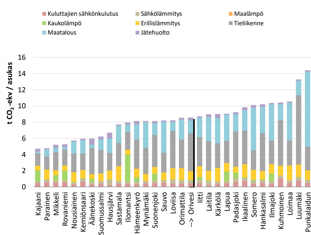
Kuva 19. Asukaskohtaisten päästöjen vertailu (ilman teollisuutta) vuonna 2019 sellaisissa CO2-raportin kunnissa, joissa on alle 25 asukasta maaneliökilometrillä.
