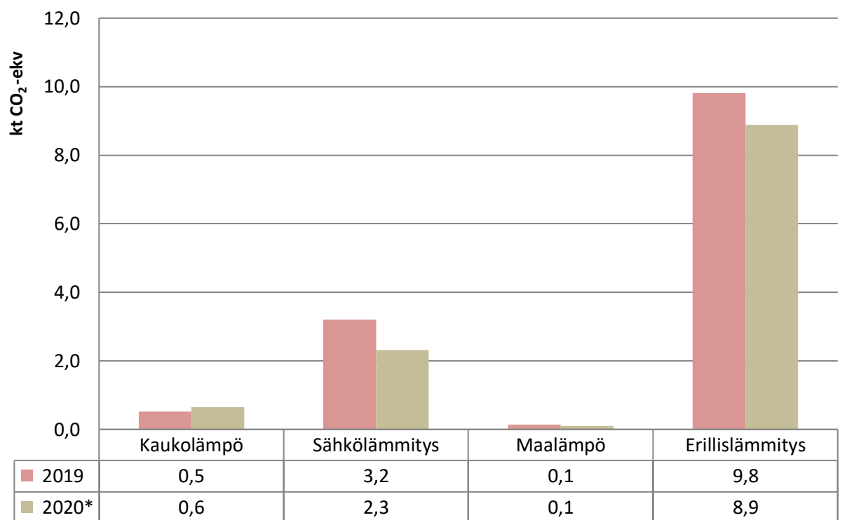
Kuva 6. Rakennusten lämmityksen päästöjen kehitys Orivedellä vuosina 2019–2020. Vuoden 2020 tieto on ennakkotieto.
