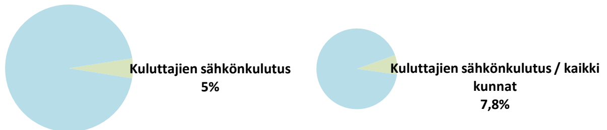
Kuva 2. Kuluttajien sähkönkulutuksen päästöjen osuus kokonaispäästöistä (ilman teollisuutta) Orivedellä ja CO2-raportin kunnissa keskimäärin vuonna 2019.
