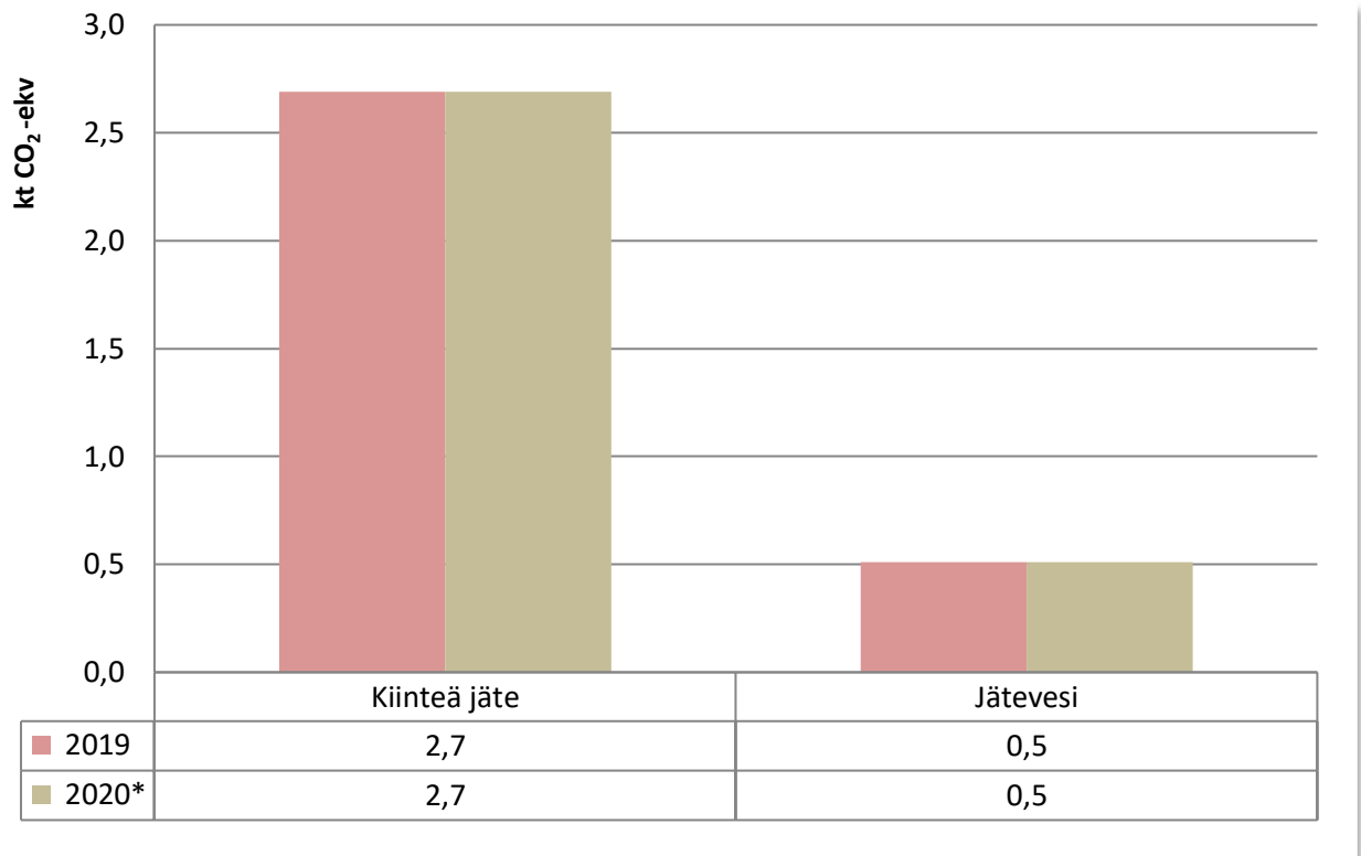
Kuva 12. Jätehuollon päästöjen kehitys Orivedellä vuosina 2019–2020. Vuoden 2020 ennakkotietona on vuoden 2019 tieto.
