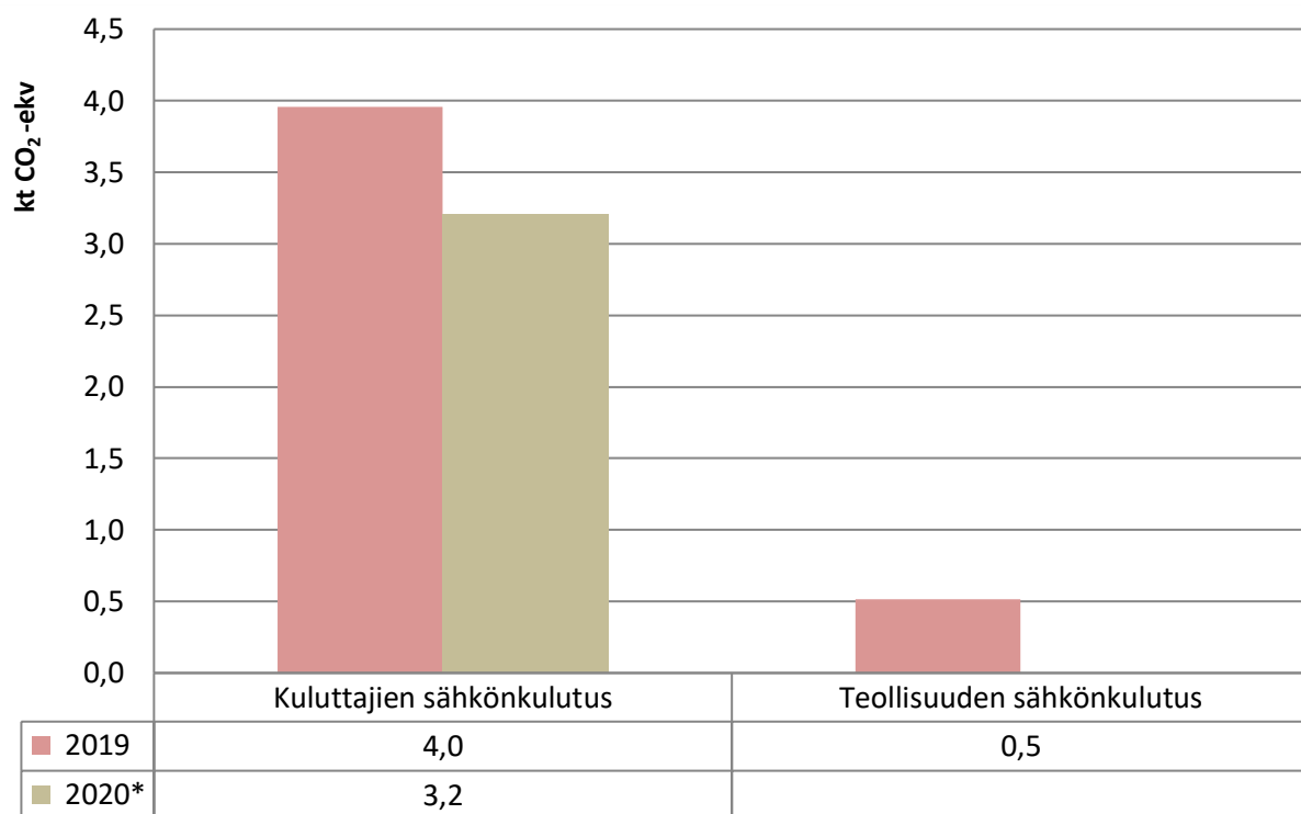
Kuva 3. Kuluttajien ja teollisuuden sähkönkulutuksen päästöjen kehitys Orivedellä vuosina 2019–2020. Vuoden 2020 tieto on ennakkotieto. Sitä ei ole esitetty teollisuuden sähkönkulutukselle.
