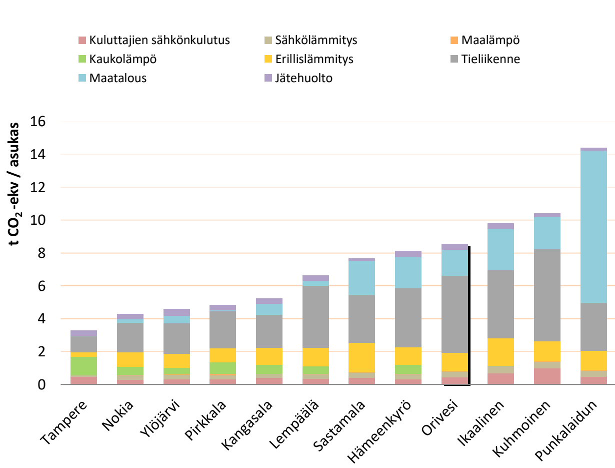
Kuva 17. CO2-raportissa mukana olevien Pirkanmaan kuntien asukaskohtaiset päästöt vuonna 2019 ilman teollisuutta.
