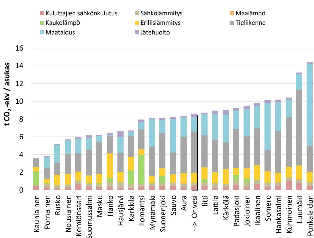
Kuva 18. CO2-raportissa mukana olevien alle 10 000 asukkaan kuntien asukaskohtaiset päästöt vuonna 2019 ilman teollisuutta.
