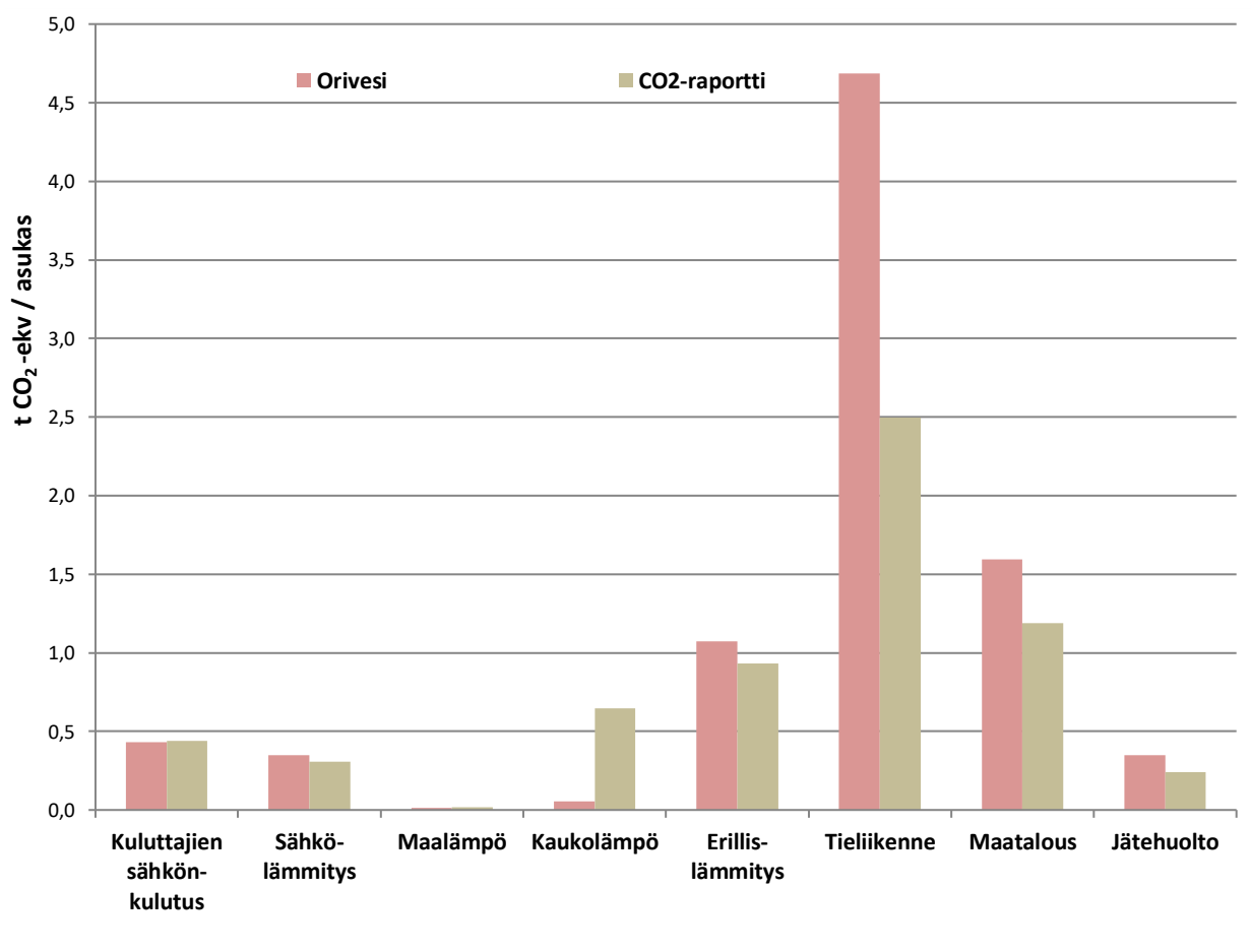
Kuva 16. Asukaskohtaisten päästöjen vertailu keskimääräiseen CO 2 -raportin kuntaan vuonna 2019.
