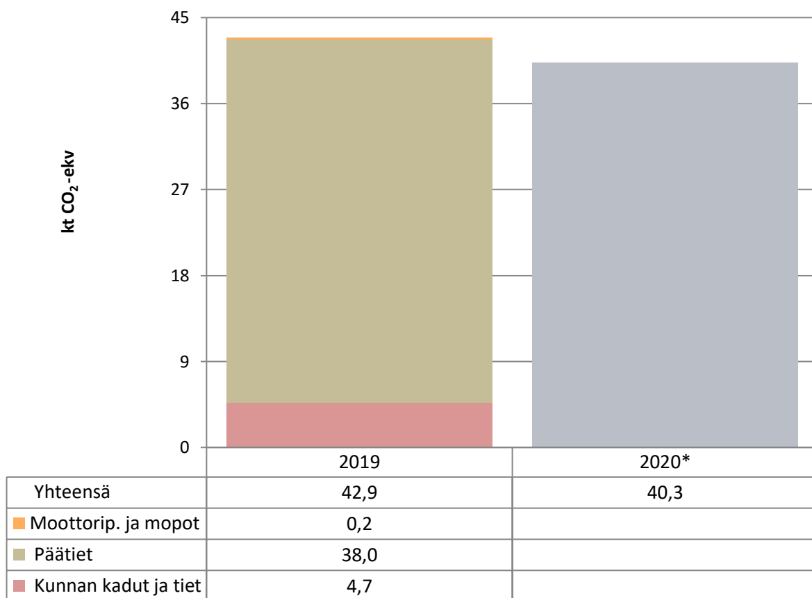
Kuva 8. Tieliikenteen päästöt Orivedellä vuosina 2019–2020. Vuoden 2020 tieto on ennakkotieto, joka perustuu liikennemäärien muutoksiin kunnan alueella.
