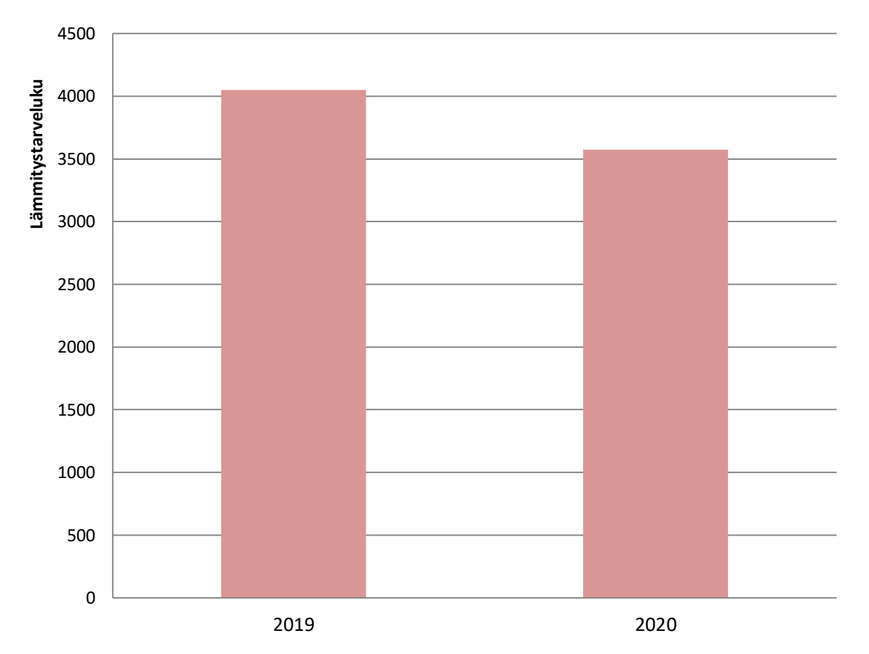
Kuva 4. Oriveden lämmitystarveluvut vuosina 2019–2020.
