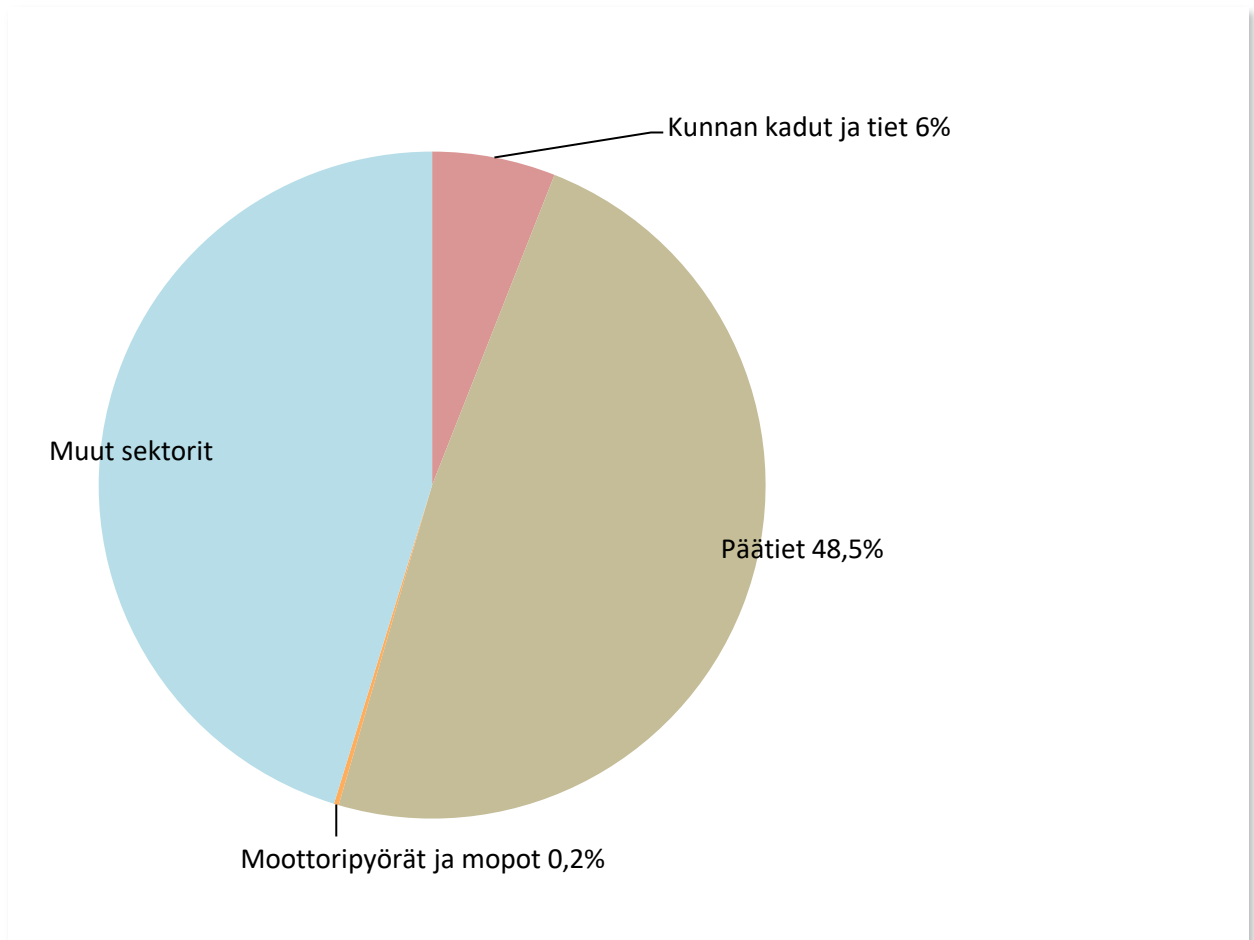
Kuva 7. Tieliikenteen päästöjen osuus kokonaispäästöistä (ilman teollisuutta) Orivedellä vuonna 2019 ja sektorin jakautuminen eri päästölähteisiin.
