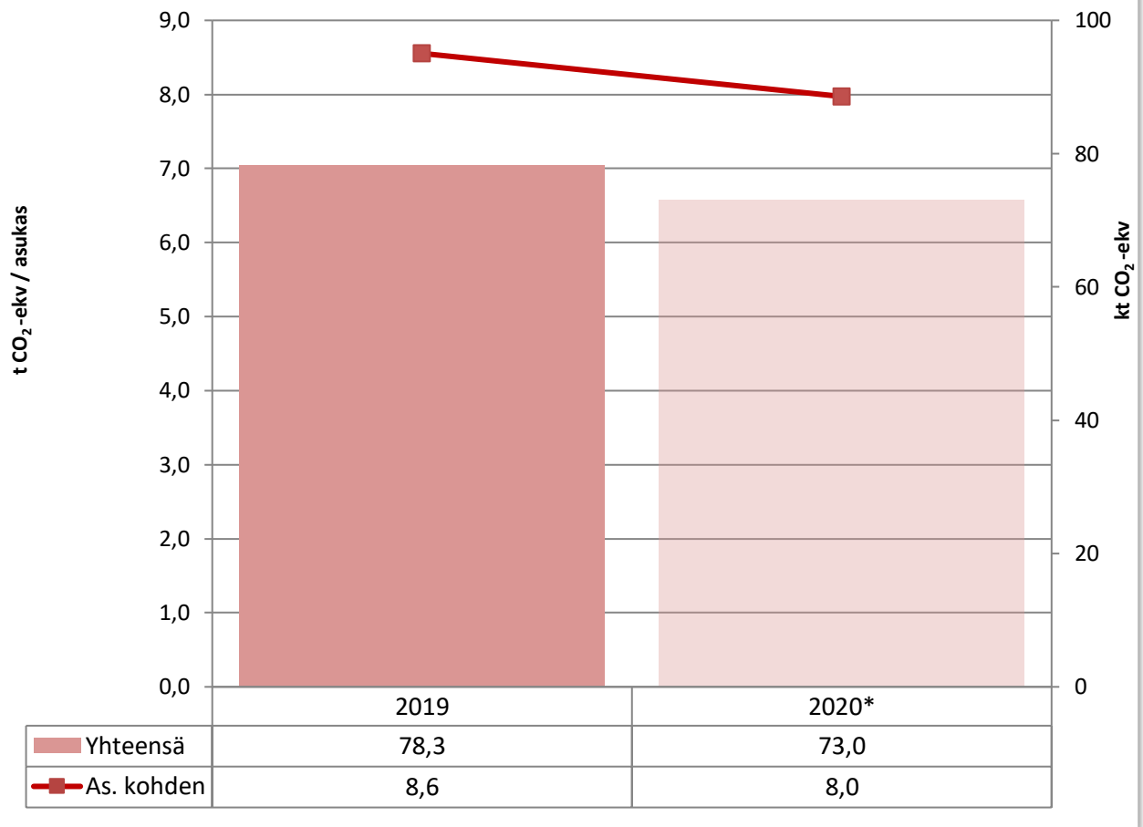
Kuva 15. Päästöt yhteensä ja asukasta kohden Orivedellä vuosina 2019–2020 ilman teollisuutta. Vuoden 2020 tieto on ennakkotieto.
